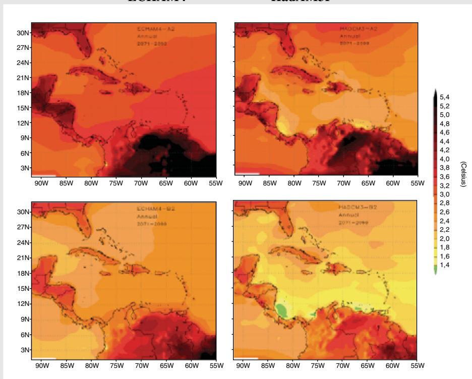
Figura 1 CAMBIOS ANUALES DE TEMPERATURA ECHAM4 HadAM3P
