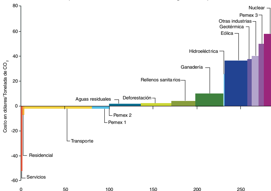
Gráfico VII.26 MÉXICO: CURVA DE COSTOS MARGINALES DE MITIGACIÓN, 2020 (En millones de toneladas de CO 2 anuales)
