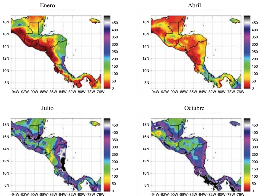
Figura IV.5 CENTROAMÉRICA: CLIMATOLOGÍA DE LA PRECIPITACIÓN, ENERO, ABRIL, JUNIO Y OCTUBRE, 1950-2000 (En milímetros)
