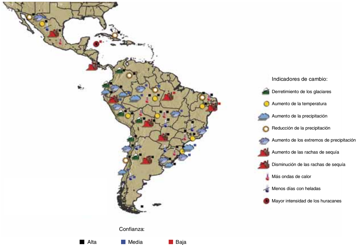
Figura IV.6 AMÉRICA LATINA Y EL CARIBE: SÍNTESIS DE LOS PATRONES DE CAMBIO CLIMÁTICO PROYECTADOS HASTA 2010 a
