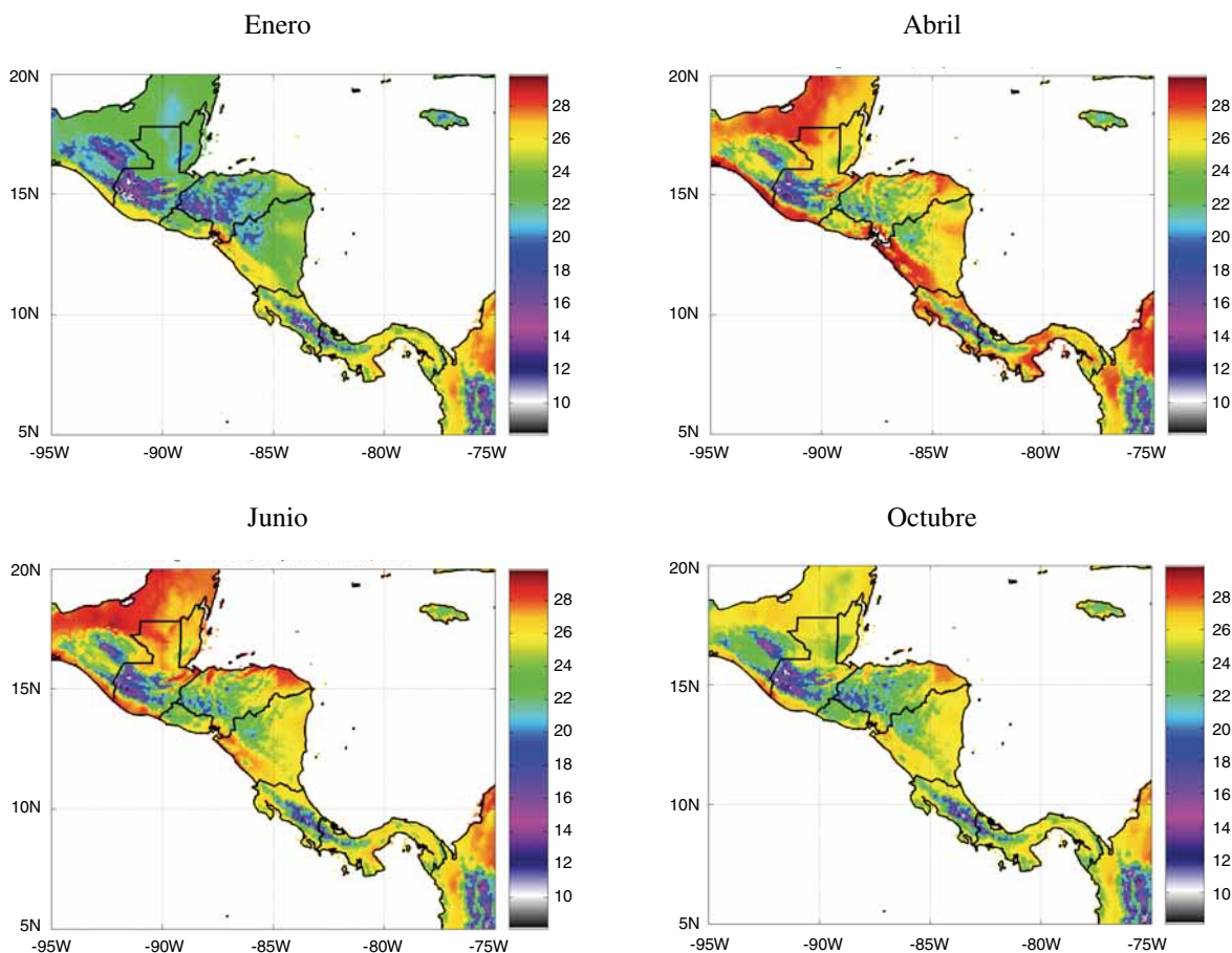
Figura IV.4 CENTROAMÉRICA: CLIMATOLOGÍA DE LA TEMPERATURA MEDIA, ENERO, ABRIL, JUNIO Y OCTUBRE, 1950-2000 (En grados centígrados)
