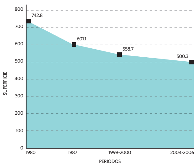
Gráfico 6.3 Retroceso de la cobertura de la superficie glaciaria (km 2 ), de la Cordillera Blanca
