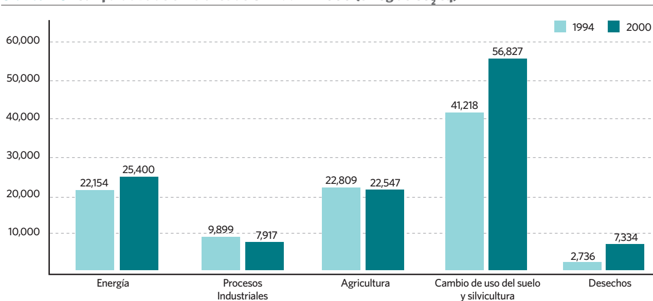
Gráfico 4.3 Comparativo de emisiones de GEI 1994 - 2000 (en Gg de CO 2 eq)
