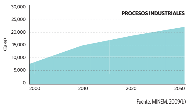
Gráfico 4.6 Proyección de emisiones de GEI en la categoría Procesos Industriales
