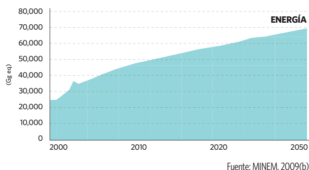
Gráfico 4.5 Proyección de emisiones de GEI en la categoría Energía
