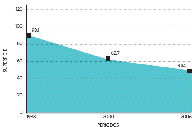
Gráfico 6.4 Retroceso de la cobertura de la superficie glaciaria (km 2 ), del Nevado Coropuna
