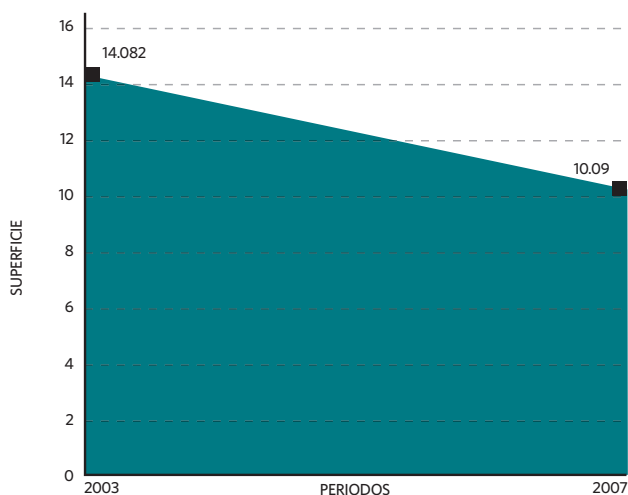
Gráfico 6.5 Retroceso de la cobertura de la superficie glaciaria (km 2 ), del Nevado Salkantay
