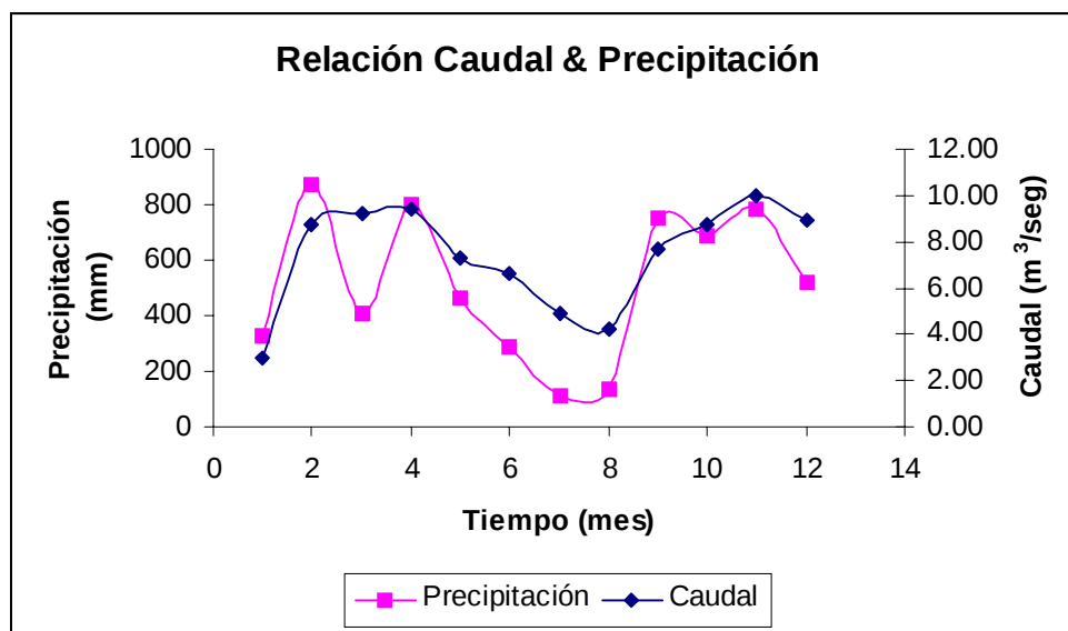
Gráfica 1. Relación entre la información mensual de precipitación (mm) y caudal observado (m³/s).
